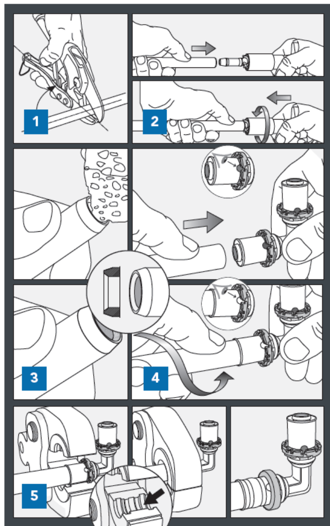
RACCORDS PROFIL TH DE 14 À 63 MM (THL POUR 32 MM)
